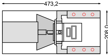
12V & 24V DC Fırçasız Servo Motor 250 W & 550 W
